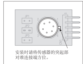
传感器安装时突起部方位
